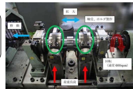
回転曲げ疲労試験装置
