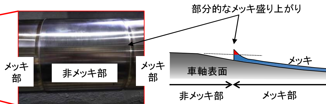
メッキ境部のメッキ盛り上がりの状態
