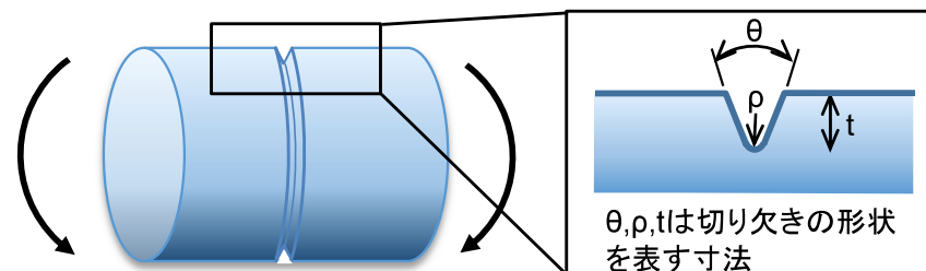
切り欠き詳細図
